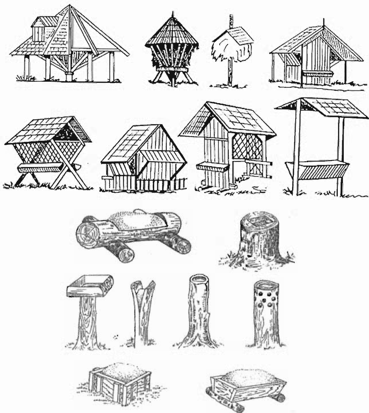
Схема 1: Схематическое изображение кормушек и солонцов для козули и оленя, рекомендуемых для сооружения
